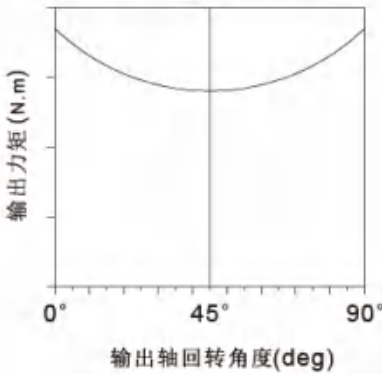
双作用输出力矩特性
