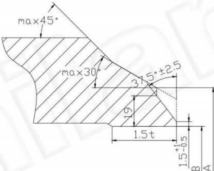
b. 管道壁厚t>22mm的焊接端
