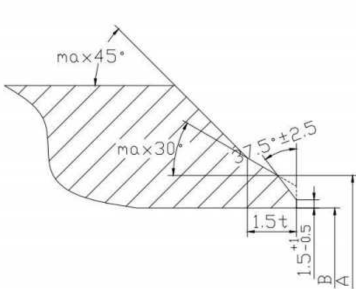
a. 管道壁厚t≤22mm的焊接端
