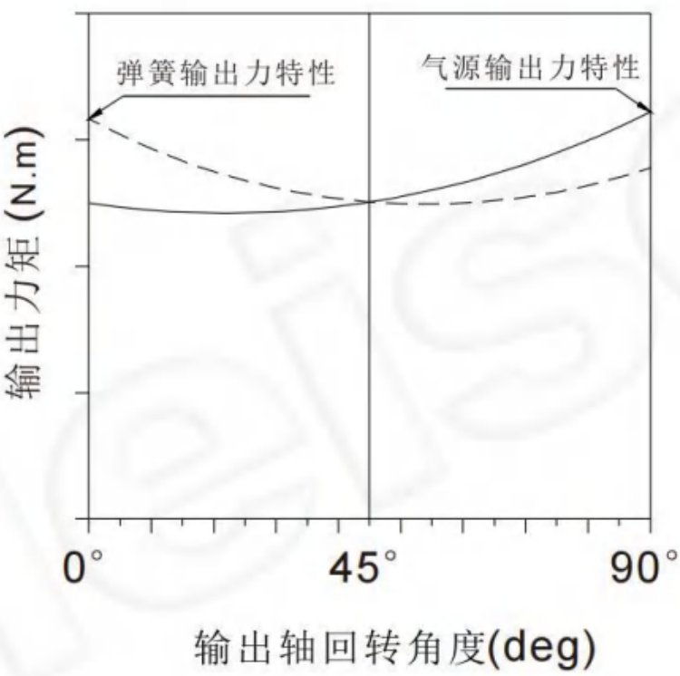
单作用输出力矩特性
