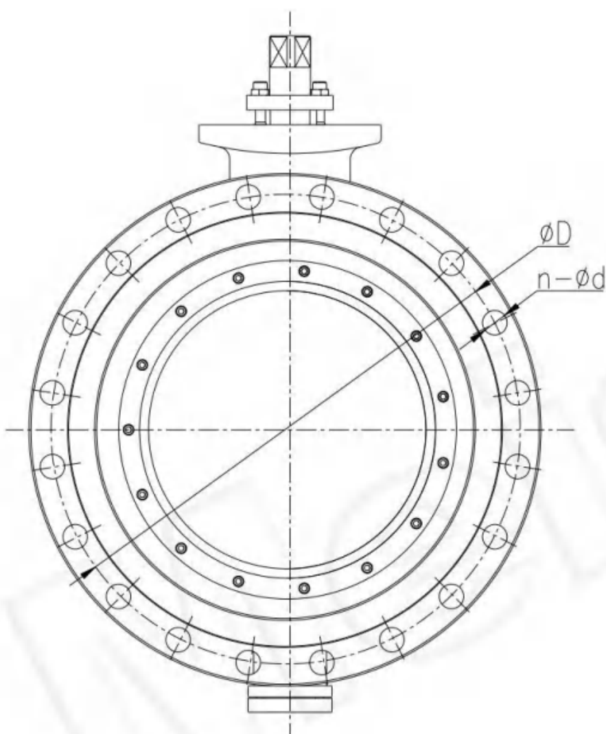
PN4.0阀体端面法兰连接尺寸
