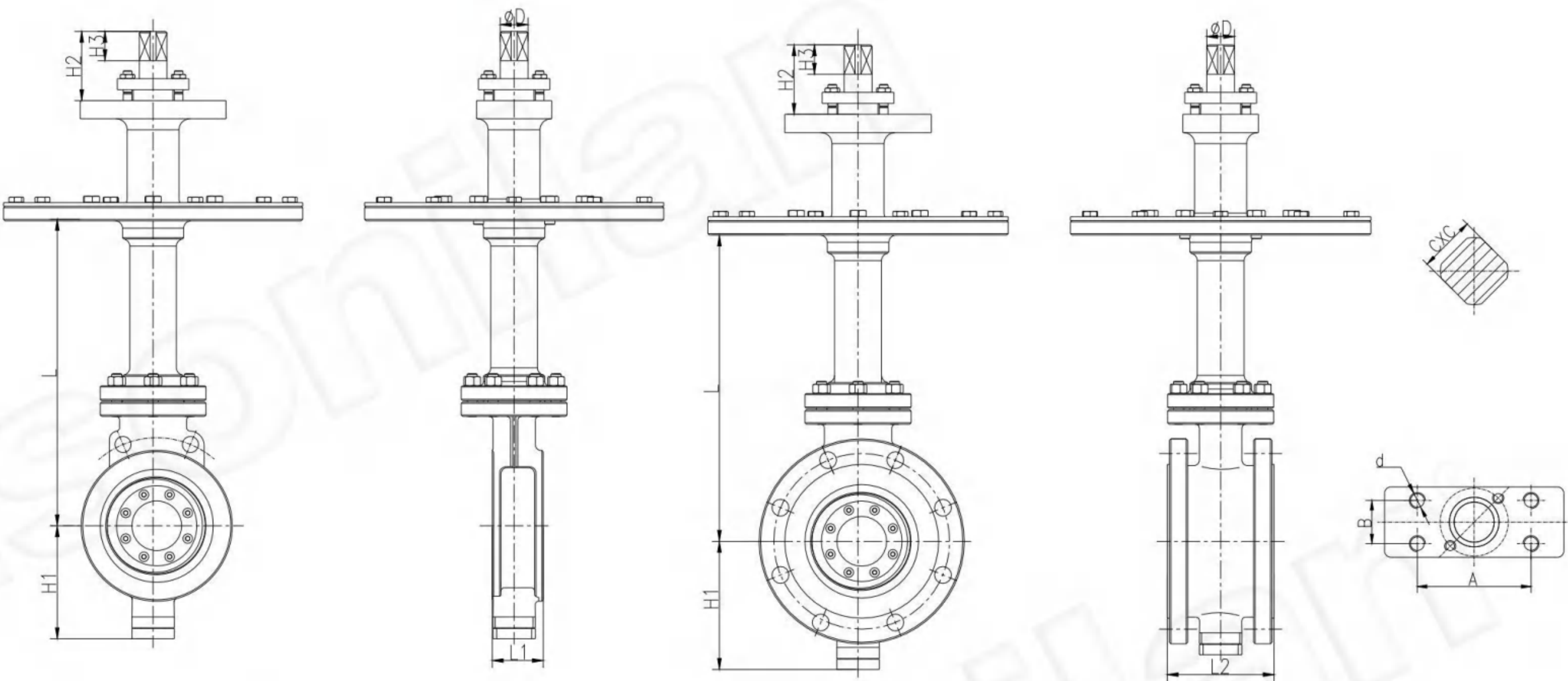
阀体结构尺寸
