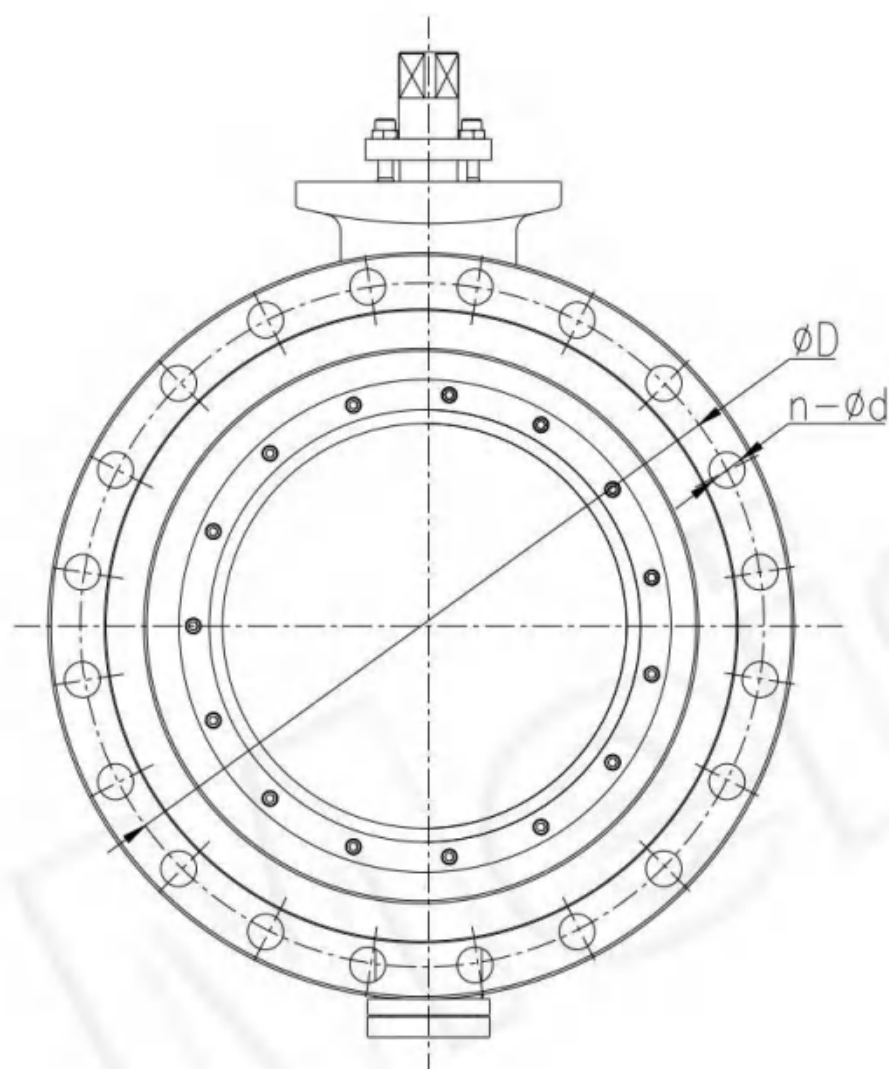
600LB阀体端面法兰连接尺寸
